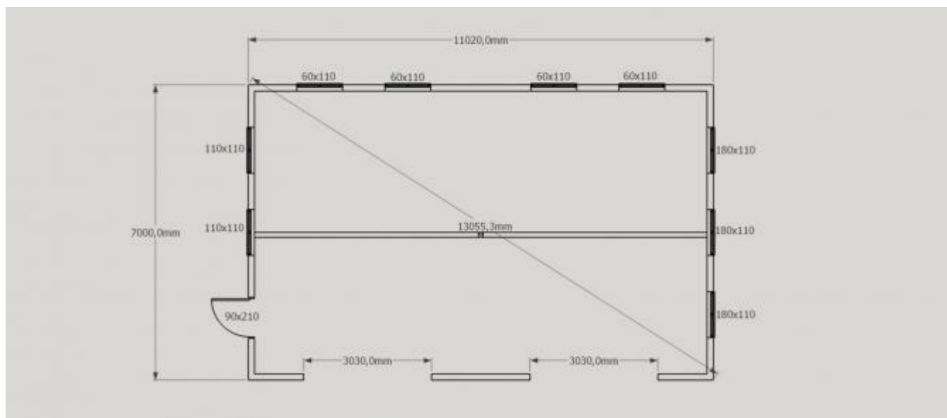
Planskisse av bygget.
