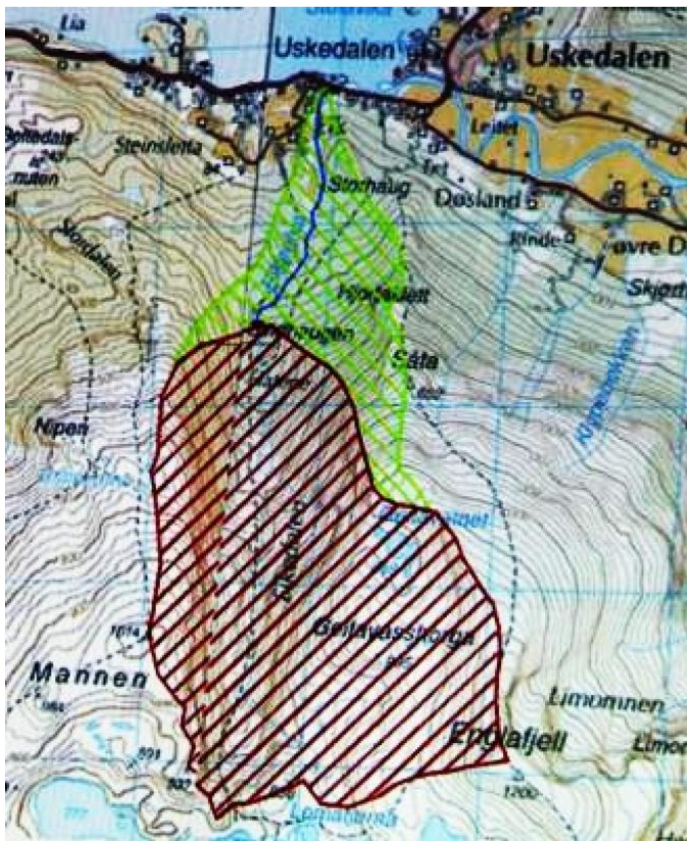
Skisse av kraftverket i Eikelva som viser nedslagsfeltet
