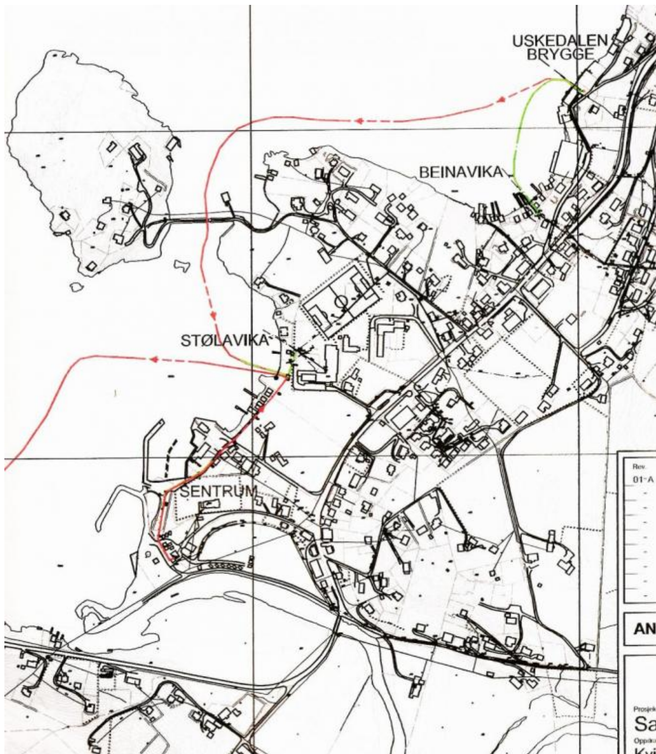
Denne skissa viser leidningane slik dei skal leggjast i dei sentrale delar av Uskedalen.
