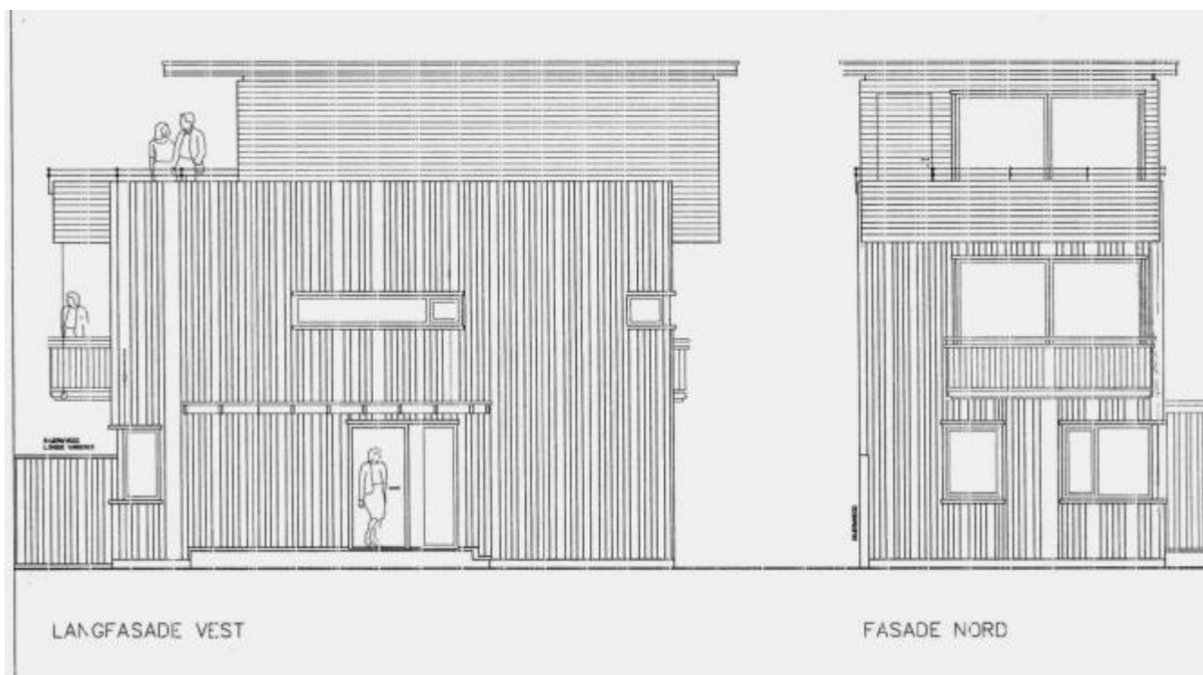
Eikeland-bustadane blir eit spanande prosjekt. Dette er to fasadar - mot vest og nord. (Teining av arkitekt Ove Grung, Bergen)
