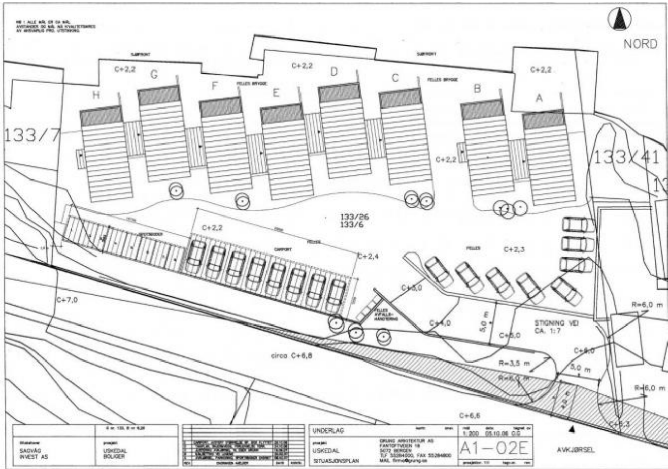
Eikelandet-prosjektet i justert utsjånad, framleis teikna av Grung Arkitektur i Bergen.
