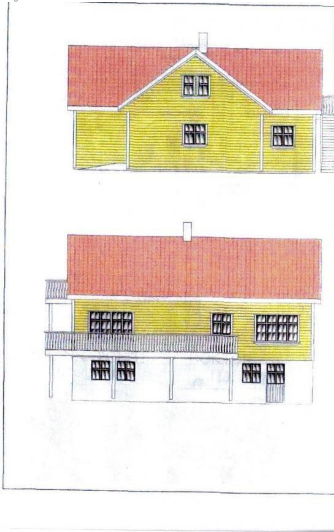
Den nye barnehagen slik han er teikna, vendt mot aust og vest.
